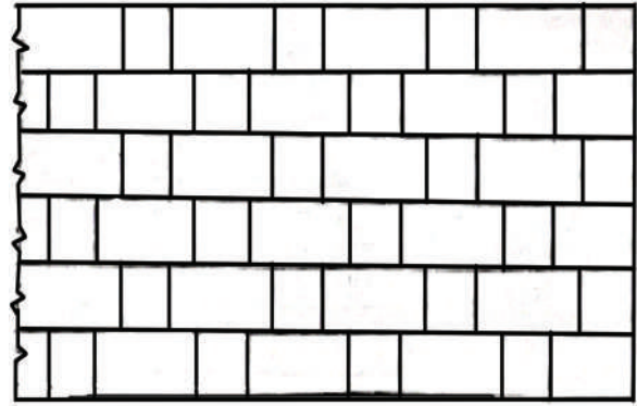
Fig. 1.16: Ashlar Fine
