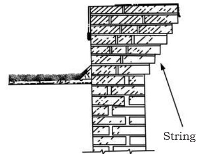
Fig. 1.4: String course
